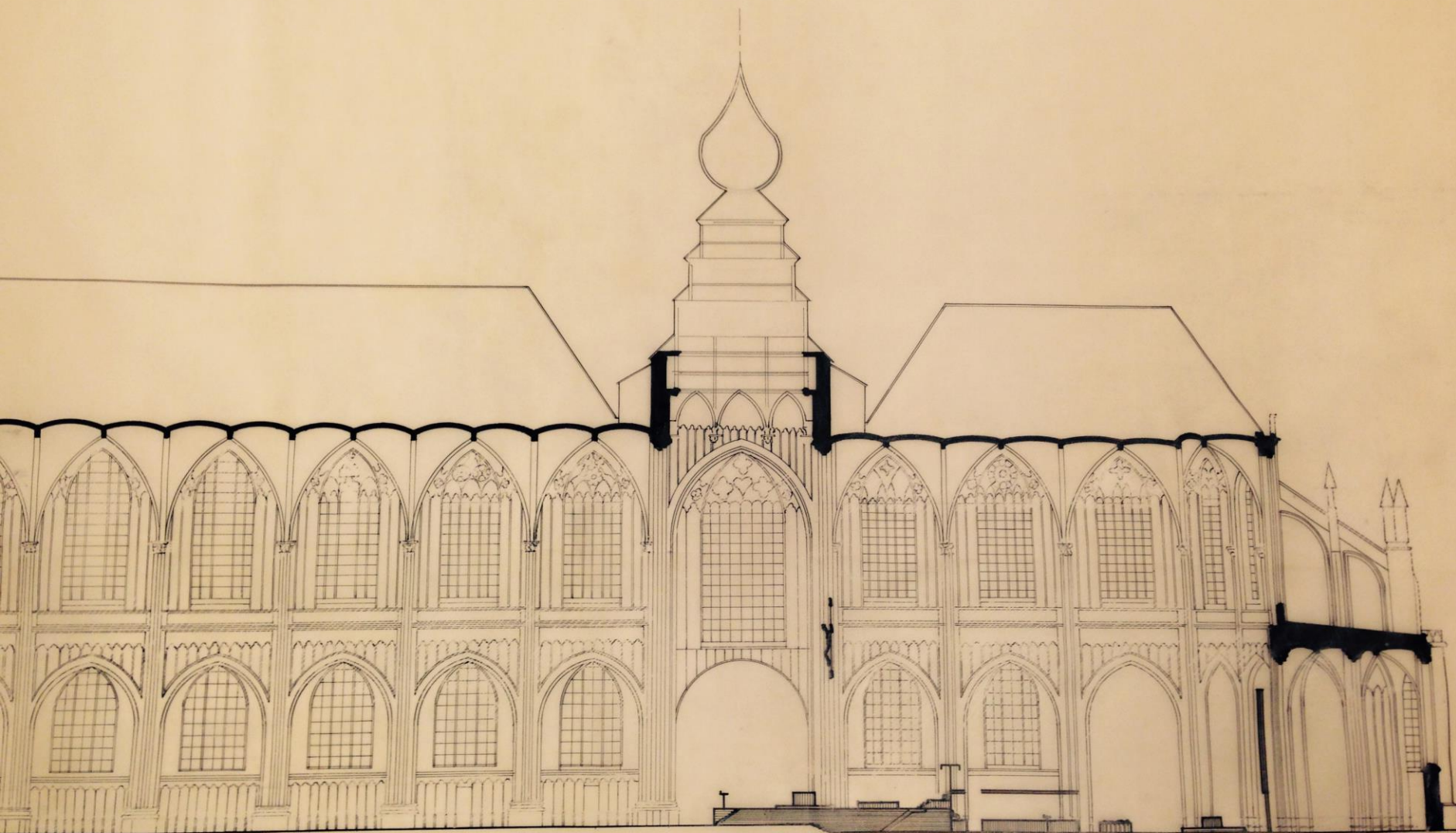
KU-Leuven, Universiteitsarchief, Fonds Raymond M. Lemaire Tekening op kalkpapier. Voorstel herinrichting koor en viering, 1963
